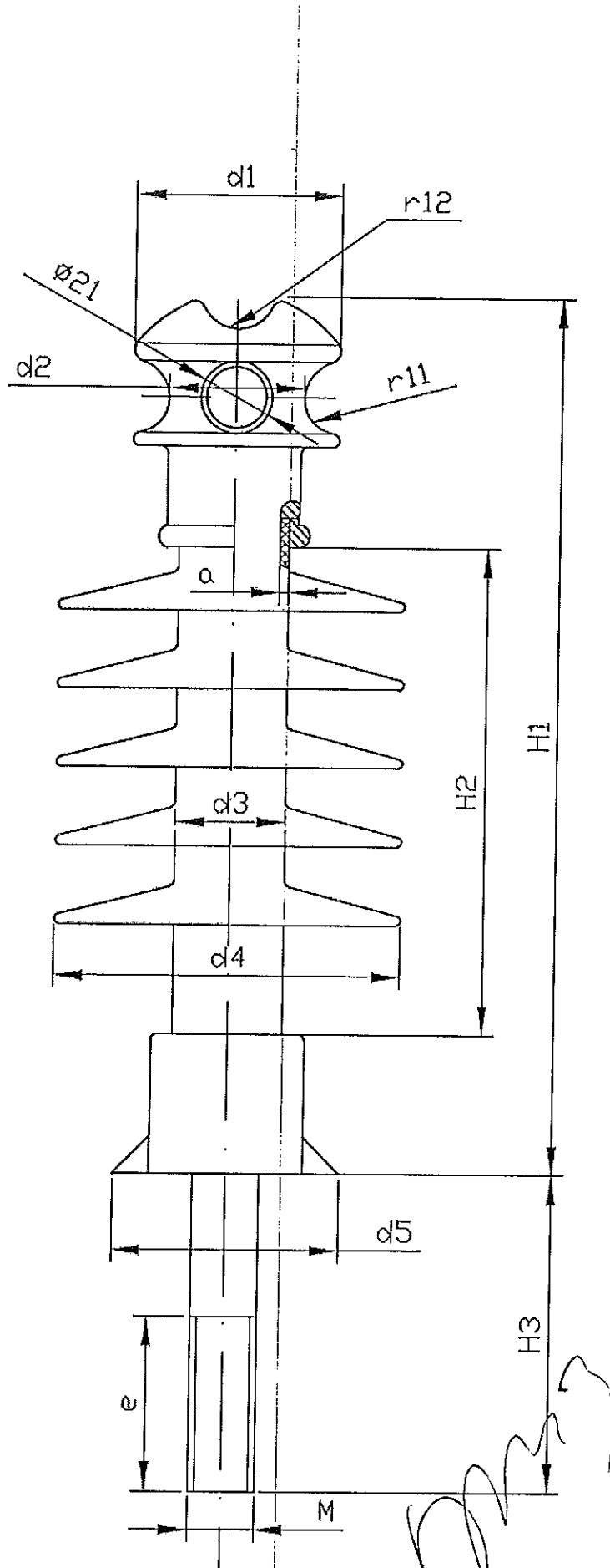
Фигура 1 - Носещ композитен изолатор 20 kV
